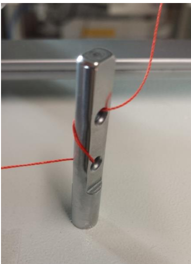
draadgeleiding garen ontwarring
