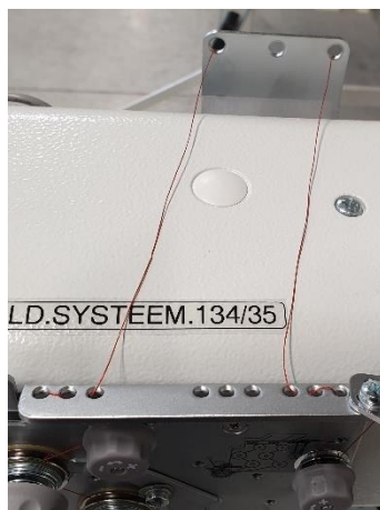
Draadgeleiding Garen ontwarren
